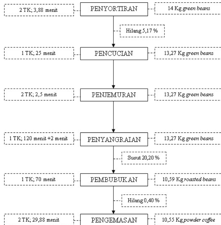
Gambar 1. Tahap Pengolahan Biji Kopi Luwak Green Beans menjadi Kopi Luwak Bubuk pada Agroindustri “Buana Putra”
