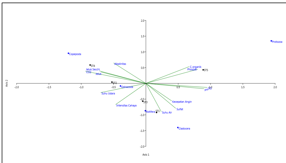
Gambar 6. Ordinasikan grup fungsional zooplankton (rotifera, cladocera, ostracoda, copepoda, dan protozoa) dengan 13 parameter fisiko-kimia (kadar oksigen terlarut, CO 2 terlarut, pH, temperatur air, temperatur udara, jeluk, jeluk Secchi, kecepatan angin, intensitas cahaya, C-organik, sulfat, fosfat) pada setiap stasiun pencuplikan menggunakan analisis korelasi kanonik (CCA).
