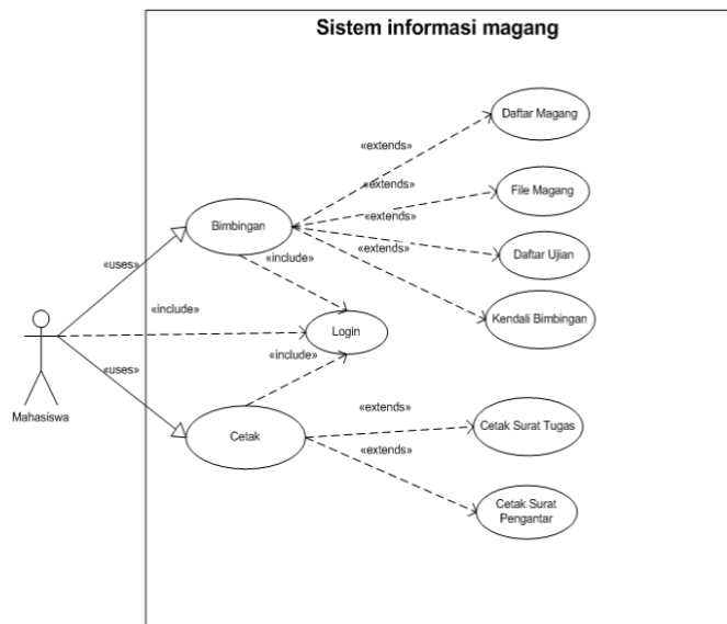
Gambar 3. Perancangan Use Case
